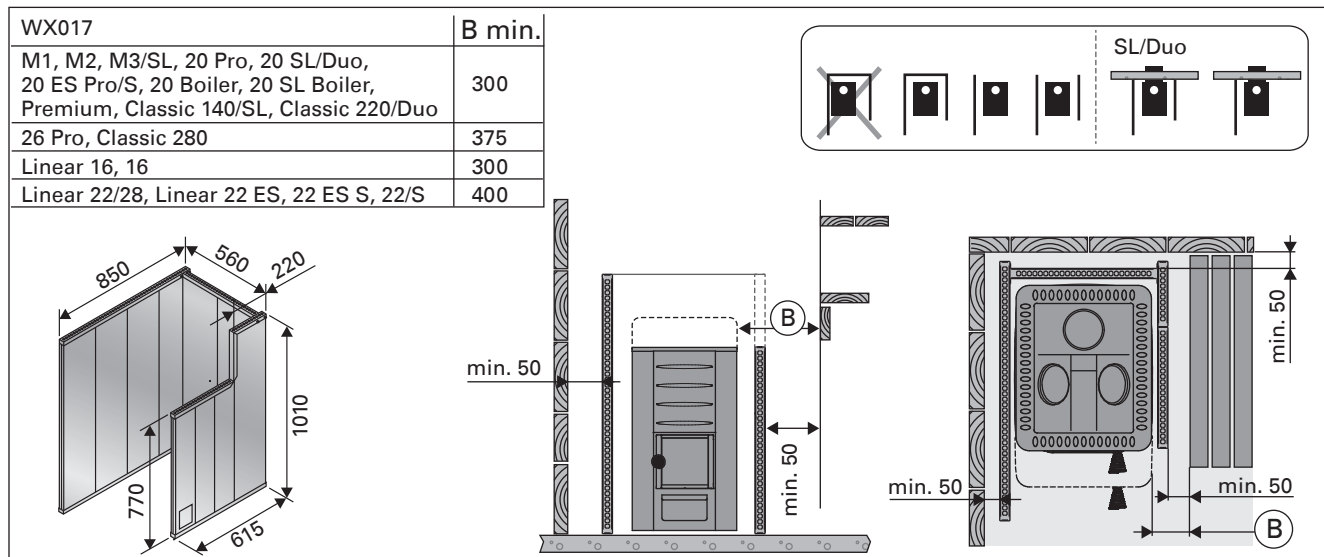
Joonis 7. Ohutuskaugused (kõik mõõtmised millimeetrites)
