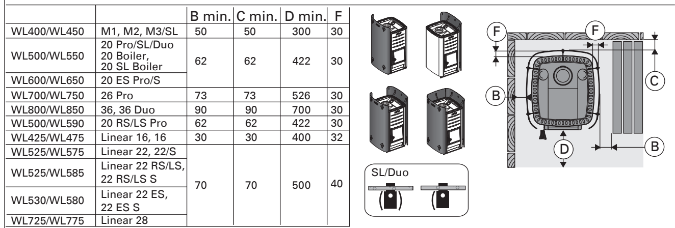
Рисунок 8. Безопасные расстояния с защитными ограждениями (все размеры приведены в миллиметрах)
