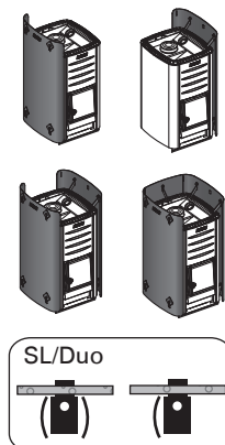
Kuva 8. Suojaetäisyydet suojaseinien kanssa (mitat millimetreinä) Bild 8. Säkerhetsavstånd med skyddsväggar (mått i millimeter)
