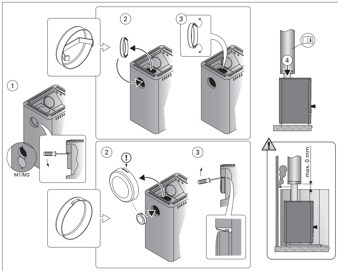
Рисунок 11. Присоединение печи к стальному дымоходу Harvia (все размеры приведены в миллиметрах) Joonis 11. Kerise ühendamise Harvia teraskorstnaga (kõik mõõdmed millimeetrites)
